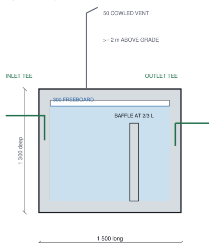
ST-01 SEPTIC TANK 1 : 40
